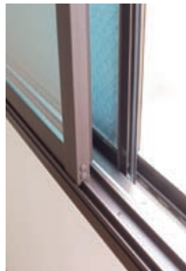
写真の外側(右側)にあるのが既存のサッシ。部屋側に内窓 インプラスを設置することで断熱性能がアップ。同時に遮音性も高くなった。
